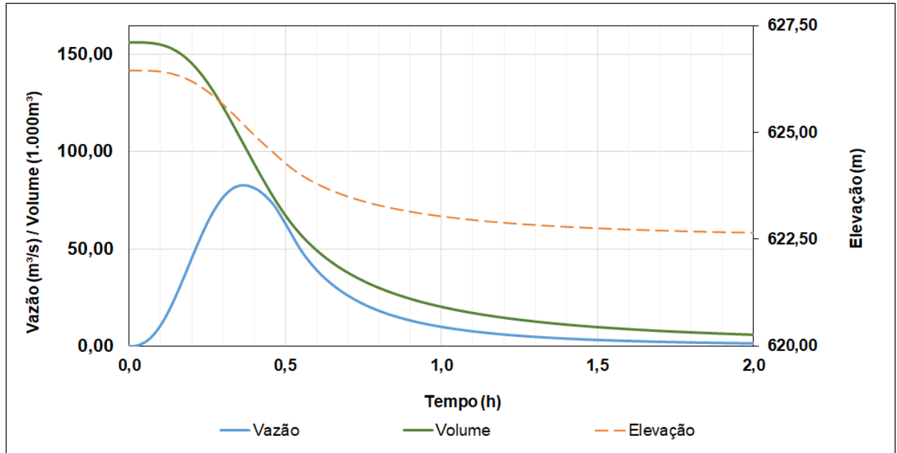
Figura 11.1 – Deplecionamento do reservatório e hidrograma de ruptura do Módulo IV.
