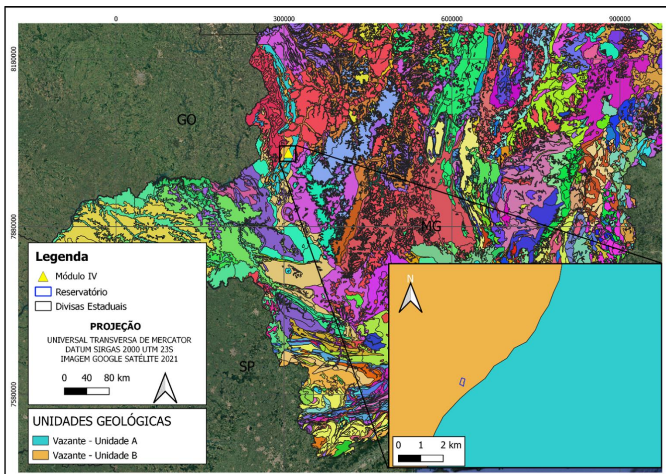
Figura 4.6 – Unidades Geológicas – Módulo IV
